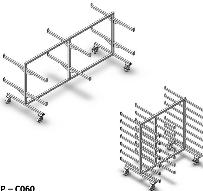
LLP – C060 Chariot de transport horizontal des profilés Dimensions en fonction des capacités souhaitées
