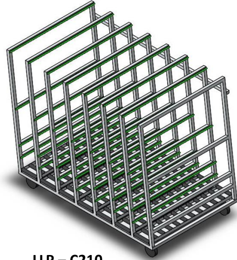
LLP – C210 Chariot de séparation de cadres
