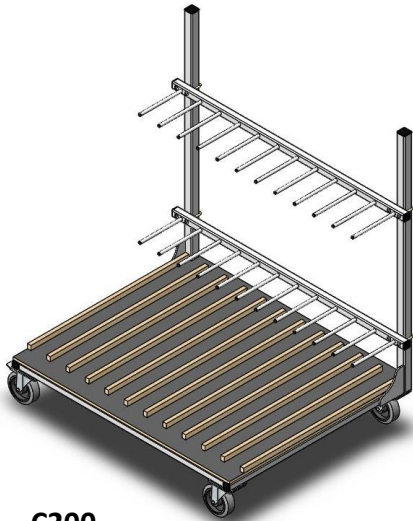
LLP – C200 Chariot de manutention pour cadres Séparateurs verticaux réglables en hauteur
