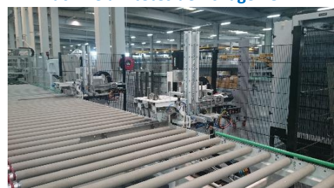
Machine à 2 têtes de fichage FOX-A2
